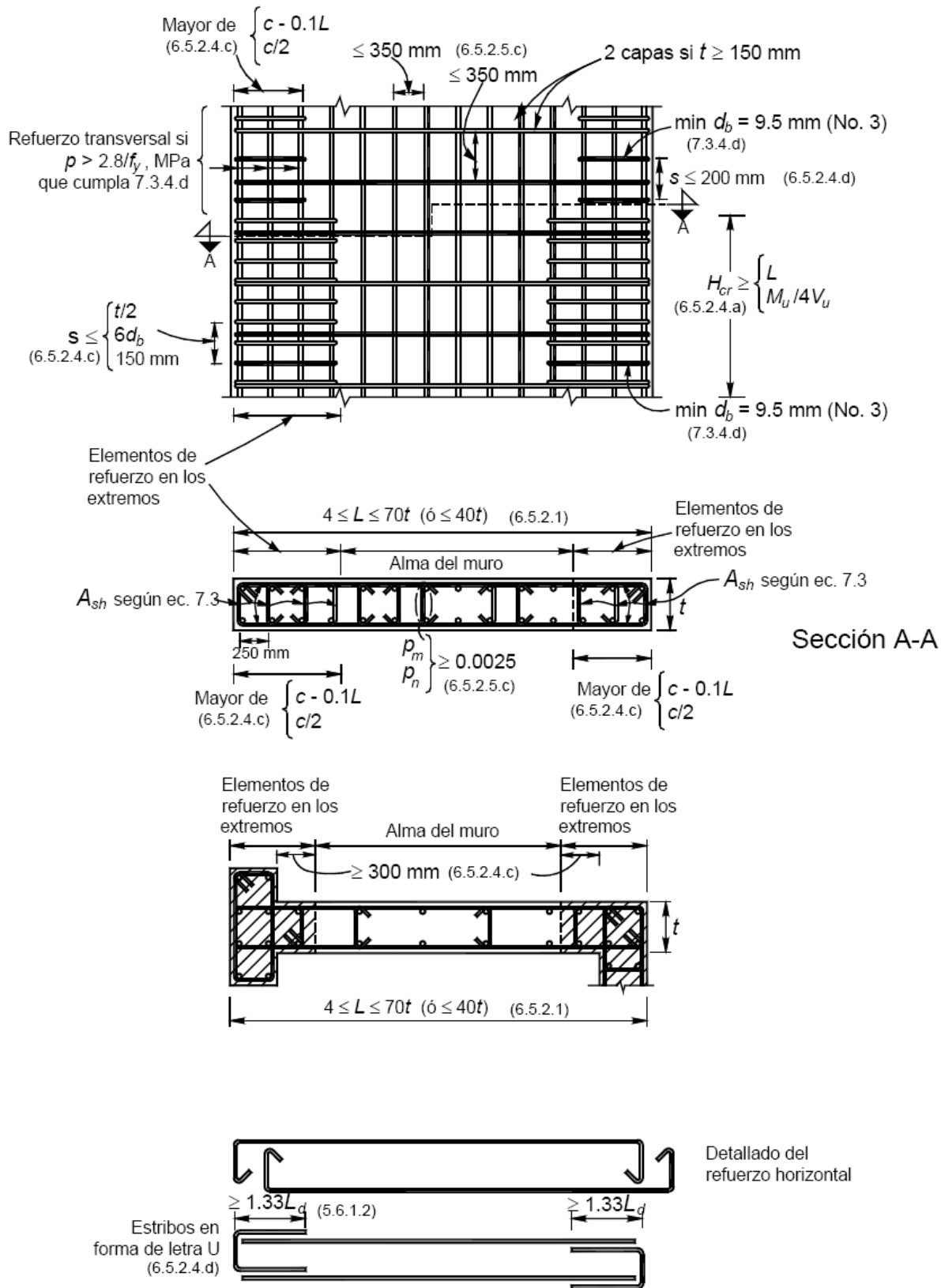
Figura 6.7 Detallado de muros
