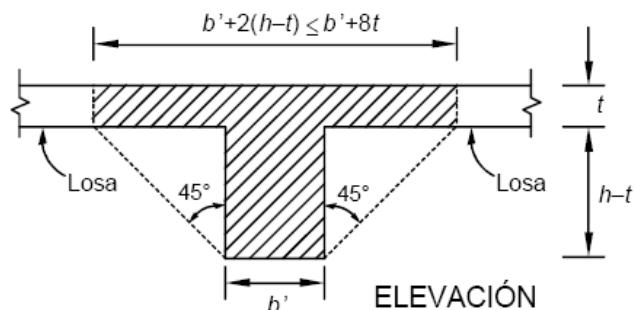
Figura 2.3 Ejemplos del tramo de losa que debe considerarse en el cálculo de A_{cp} y p_{cp}
