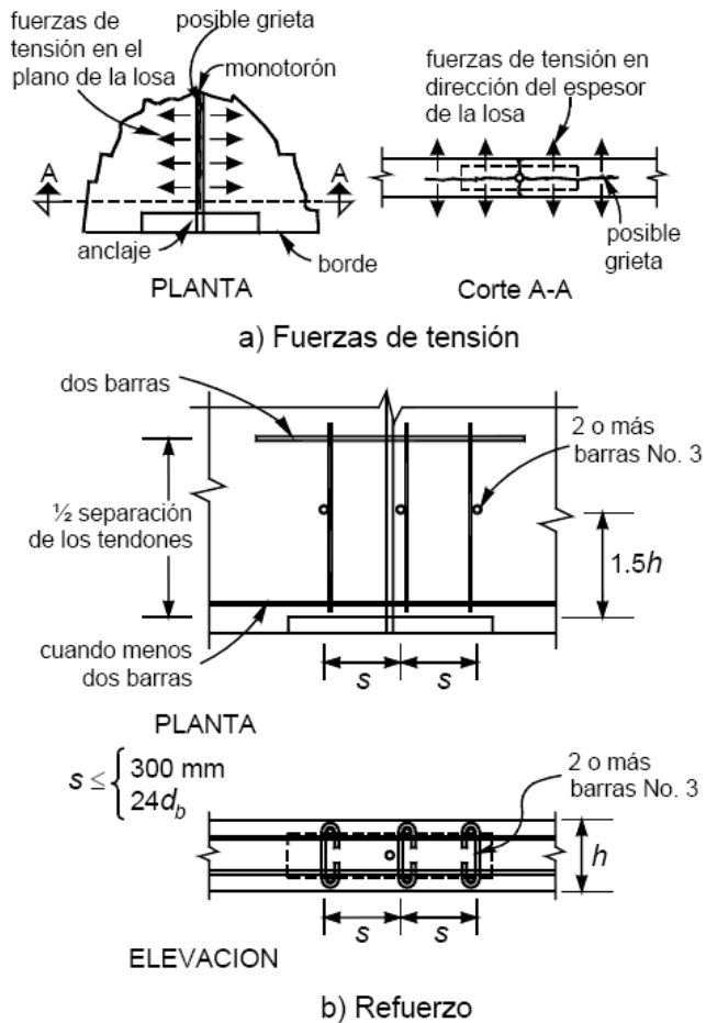
Figura 9.3 Refuerzo en la zona de anclaje
