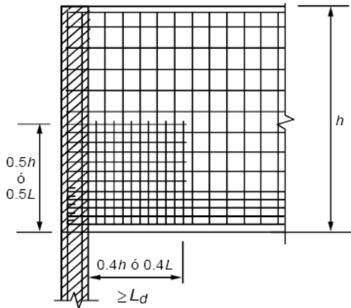
Figura 6.4 Refuerzo en una zona de apoyo indirecto
