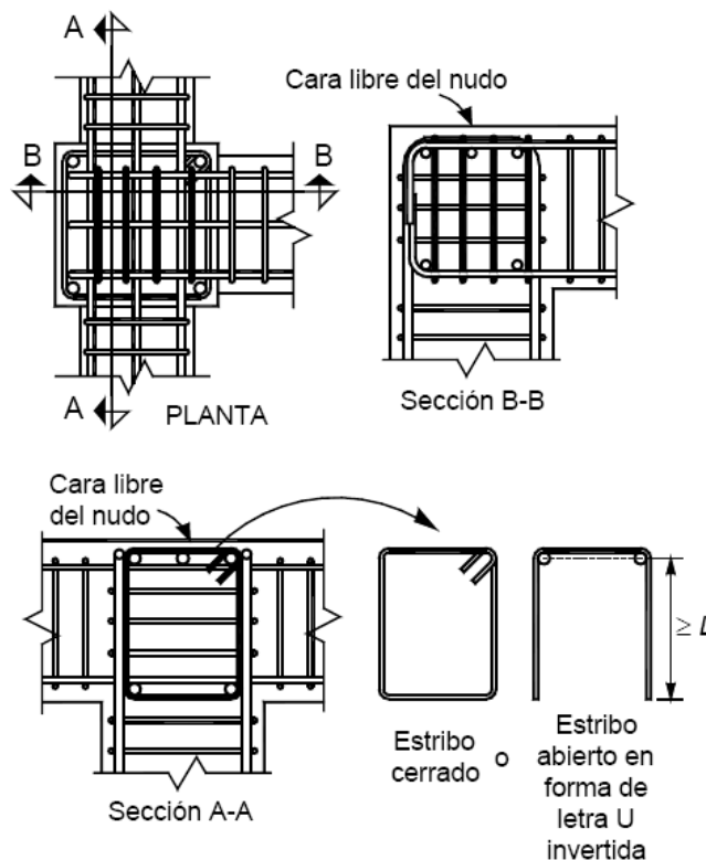
Figura 7.5 Refuerzo transversal vertical en uniones viga – columna
