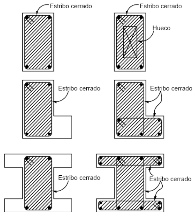
Figura 2.5 Definición del área A_{oh} (zonas sombreadas)
